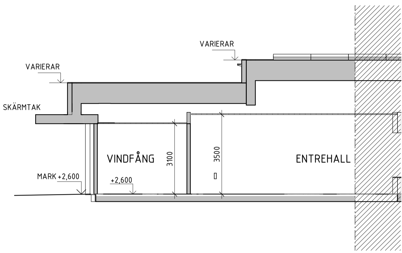
SEKTION 2-2, DEL 1
