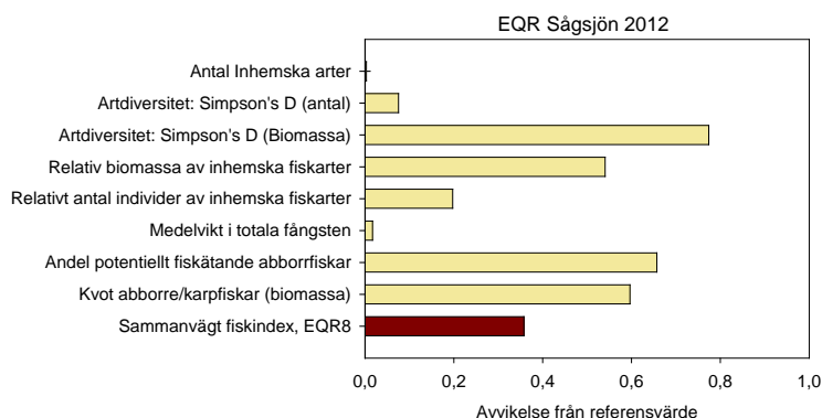
Fig. 3. Klassificering av provfiskeresultatet enligt EQR8 vid provfisket 2012 i Sågsjön. Figuren anger p-värden för de olika variablerna som sammanvägs i fiskindexet (EQR8). Avvikelsen från referensvärdet minskar då p närmar sig 1. Enligt det sammanvägda fiskindexet EQR8 har Sågsjön måttlig ekologisk status (se Tab. 2 för statusklassificeringar).
