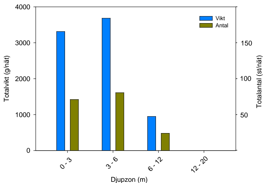
Fig. 5. Genomsnittlig totalvikt (blå staplar, vänster Y-axel) och genomsnittligt totalantal (gröna staplar, höger Y-axel) per djupzon under provfisket i Sågsjön. Totalvikten och totalantalet fångade individer var som högst i djupzonen 3-6 meter följt tätt följd av djupzonen 0-3 meter. Vid 6-12 meters djup sjönk fångsten och under 12 meter fångades ingen fisk. Denna fångstfördelning är typisk för en övergödd sjö med dåliga syrgasförhållanden under språngskiktet sommartid.
