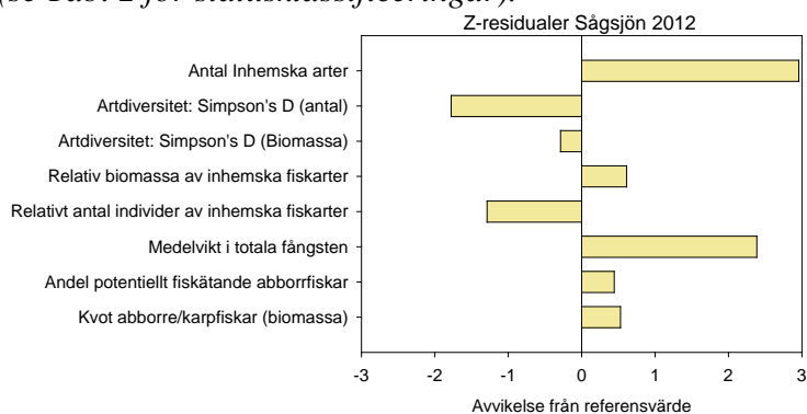
Fig. 4. Z-värdena visar om avvikelserna för respektive indikator är högre (större än 0) eller lägre än referensvärdet (mindre än 0). Om Z-värdet är noll överensstämmer provfiskeresultatet med referensvärdet. I Sågsjön finns två statistiskt signifikanta avvikelser vilka är att andelen inhemiska arter och medelvikten är högre än väntat. Denna avvikelse indikerar på att Sågsjön är påverkad av övergödning (Tab. 3).
